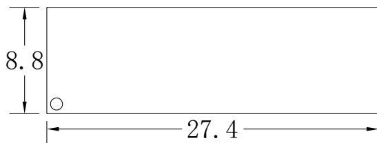
外形尺寸及管脚定义图: (标注单位: 毫米/英寸)
