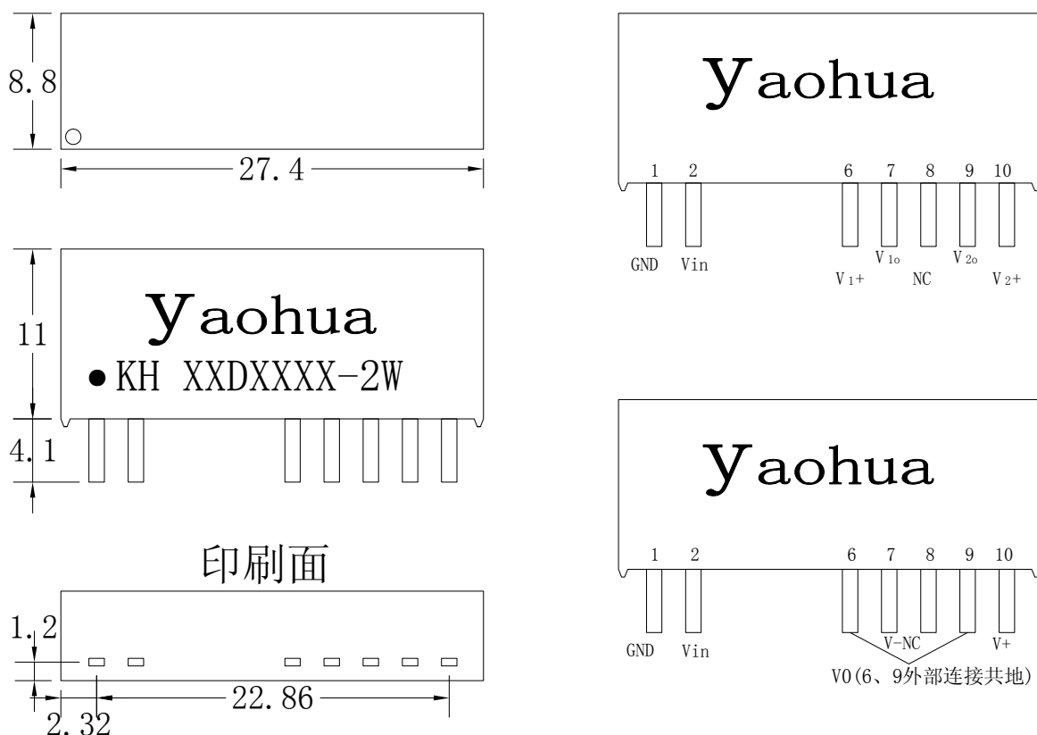
外形尺寸及管脚定义图: (标注单位: 毫米/英寸)
